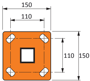
Detalj av bottenplatta bomstöd. Monteras med 4 st M10 expanderbult.
