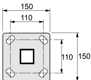
Detalj av bottenplatta bomarmstöd Monteras med 4×M10 expanderbult
