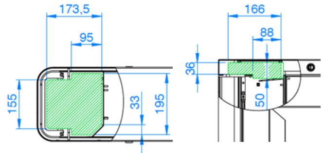
Utrymme för integration av läsare (kit som tillval).
