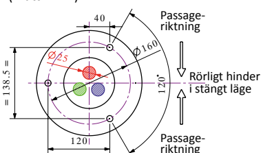
Detalj infästning mot golv (mått i mm)
