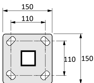
Detalj av bottenplatta bomarmsstöd. Monteras med 4xM10 expanderbult.
